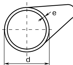
Сортамент труб ИКАПЛАСТ из полиэтилена по ГОСТ 18599-2001
