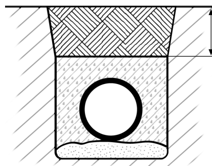
Рис. 4.1.5. Окончательная засыпка траншеи
